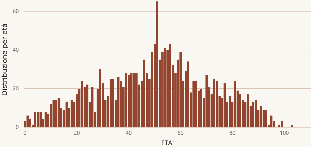
Distribuzione dell'età relativa ai Nuovi Positivi
