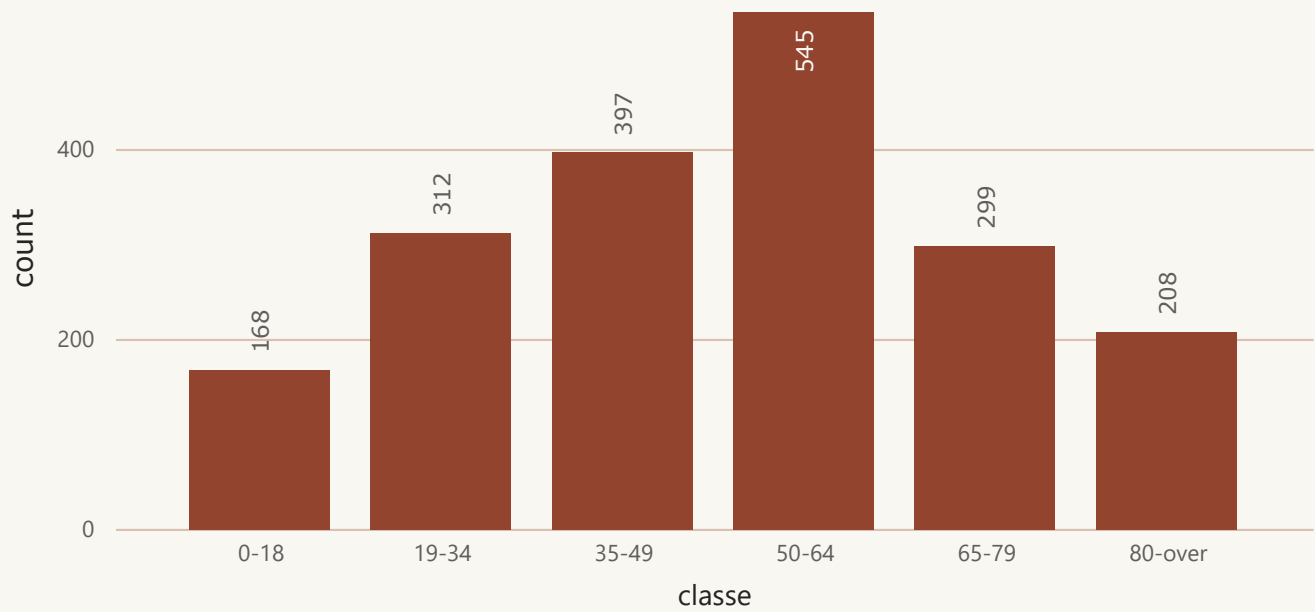
Distribuzione dei Nuovi Positivi per classe di età
