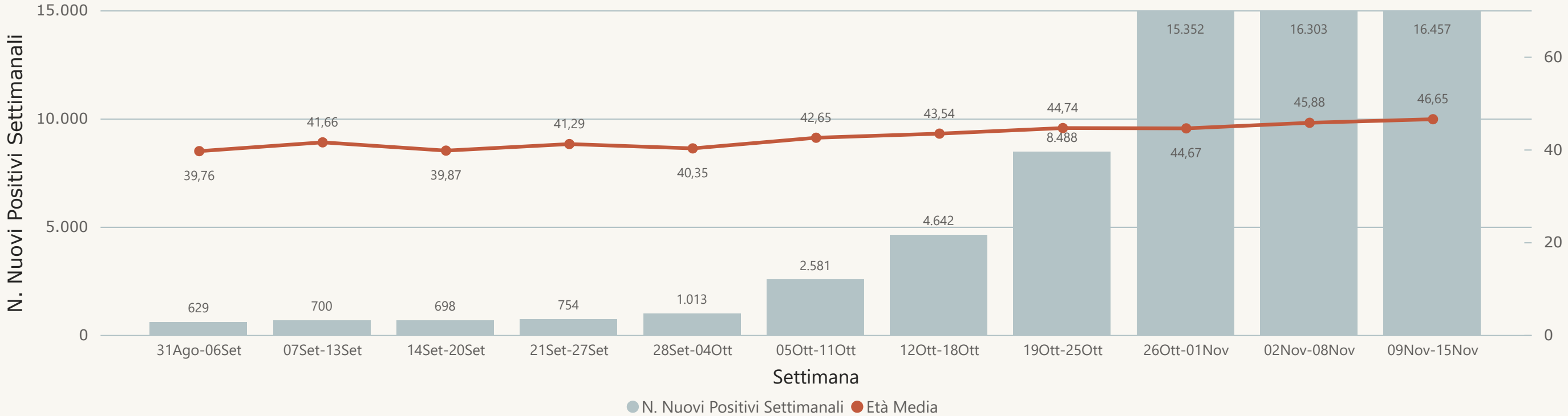
N. Nuovi Positivi ed Età Media per Settimana
