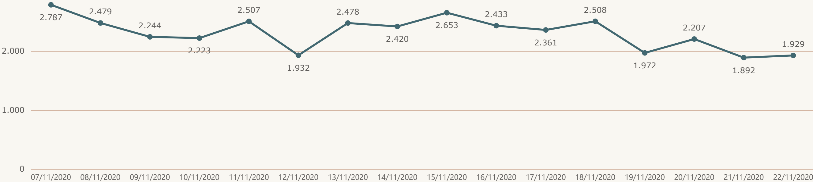
Andamento Nuovi Positivi
